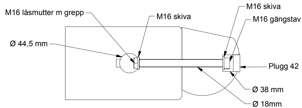
A-A (1 : 5)
